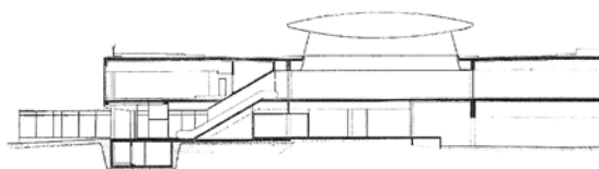
Tvärsnitt av affärshuset med arkader, gånggata och övertäckt torg.
